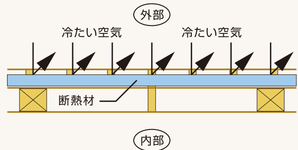
外張断熱工法(SHS工法)
