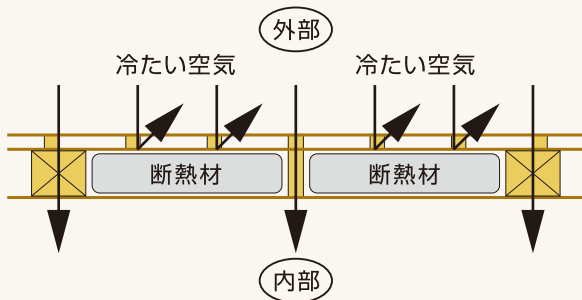
充填断熱工法(在来の工法)
